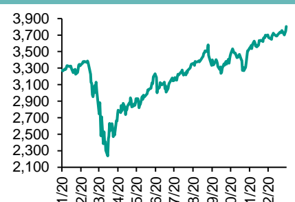
標普500走勢圖
